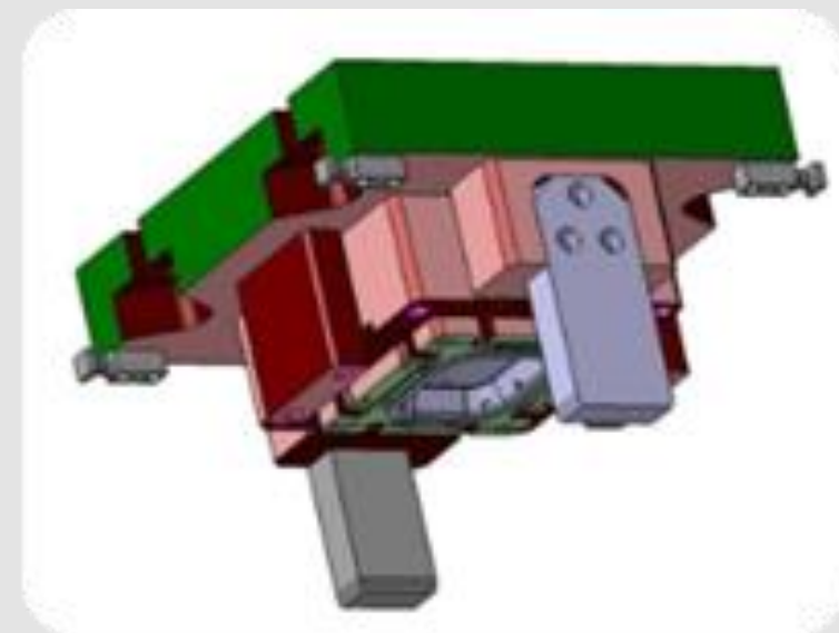
Primjer konstrukcije alata za duboko izvlačenje
