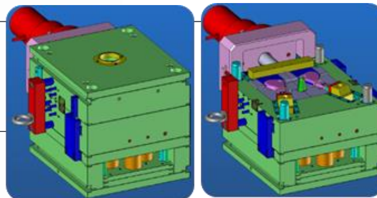
Primjer konstrukcije za zamak-cink
