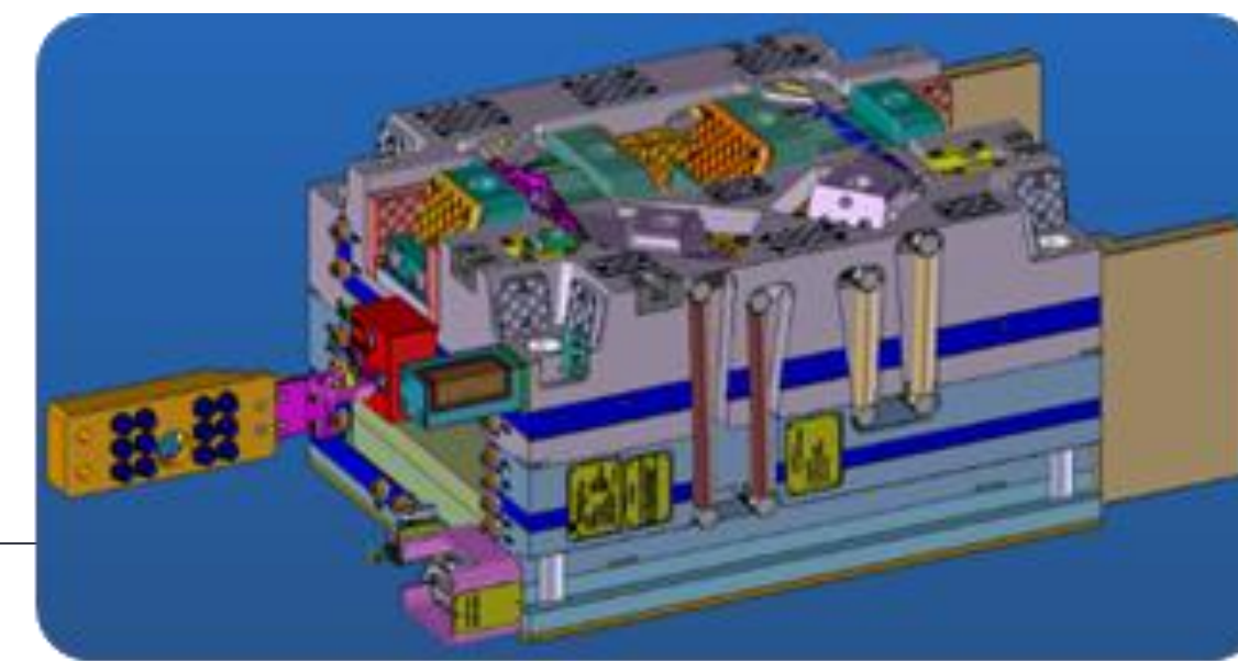
Primjer konstrukcije za plastični komad
